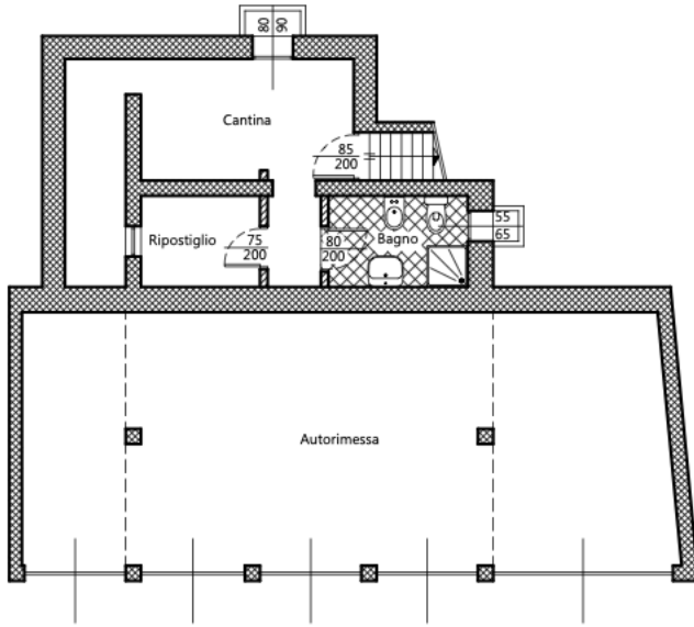
PIANO TERRA (SEMINTERRATO)
