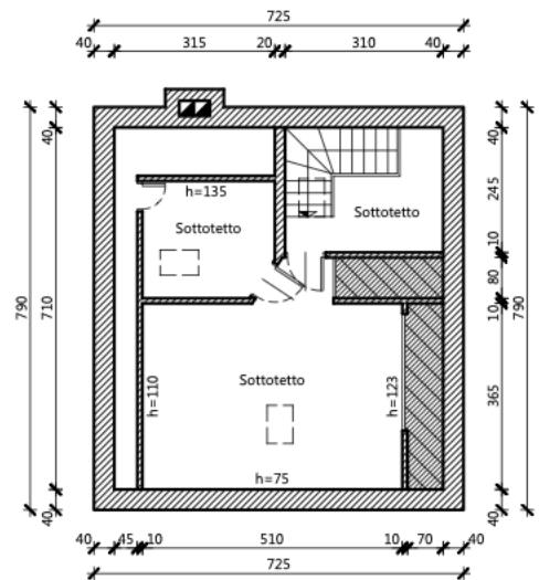
PIANO TERZO (SOTTOTETTO)
