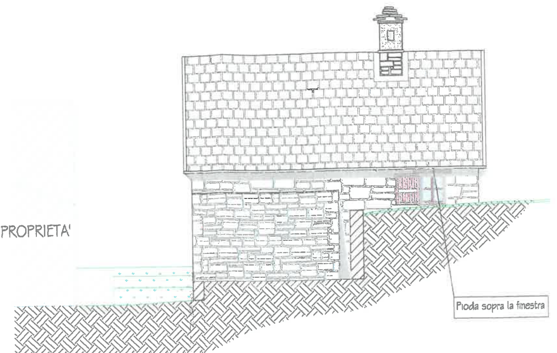
PROSPETTO NORD
