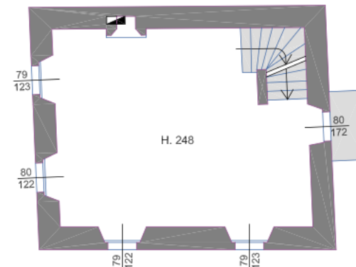
PIANTA PIANO PRIMO Scala 1:100
