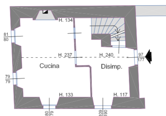
PIANTA PIANO TERRENO Scala 1:100
