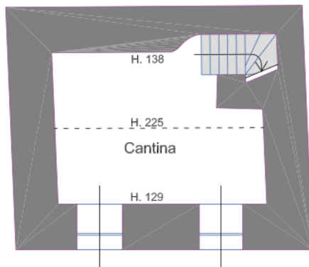
PIANTA PIANO INTERRATO Scala 1:100
