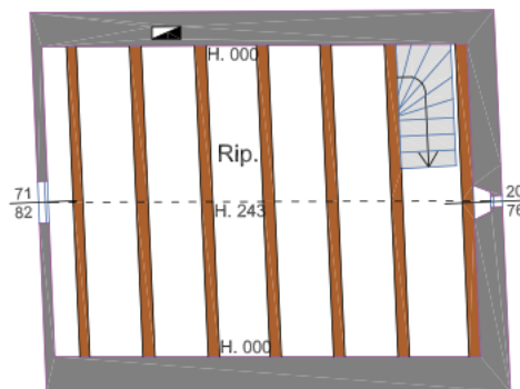
PIANTA PIANO TERZO Scala 1:100
