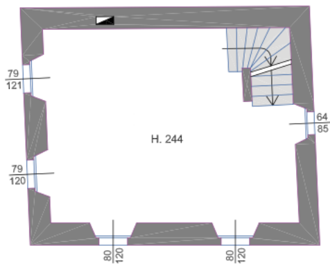
PIANTA PIANO SECONDO Scala 1:100
