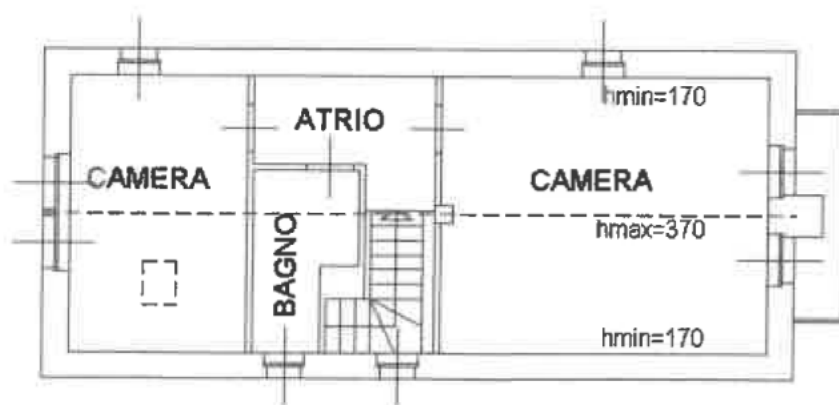
PIANO PRIMO h_m=270
