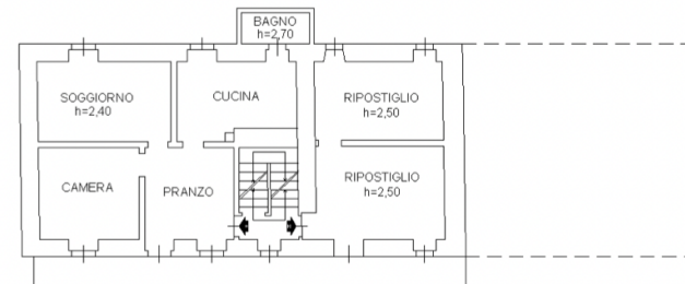
PIANO SECONDO
